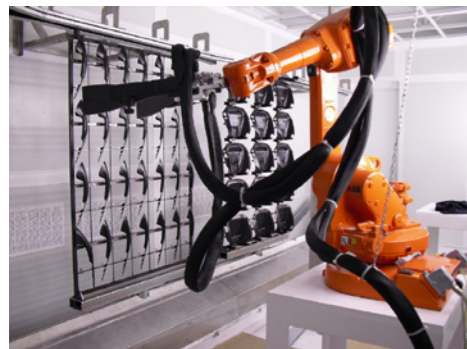
Čištění plastových dílů před lakováním aplikací Cryosnow za pomoci robota
